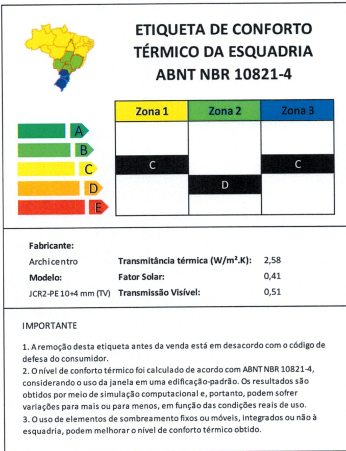
Figura – Classes de desempenho térmico da amostra TE-016 (a) persiana recolhida; (b) persiana estendida
