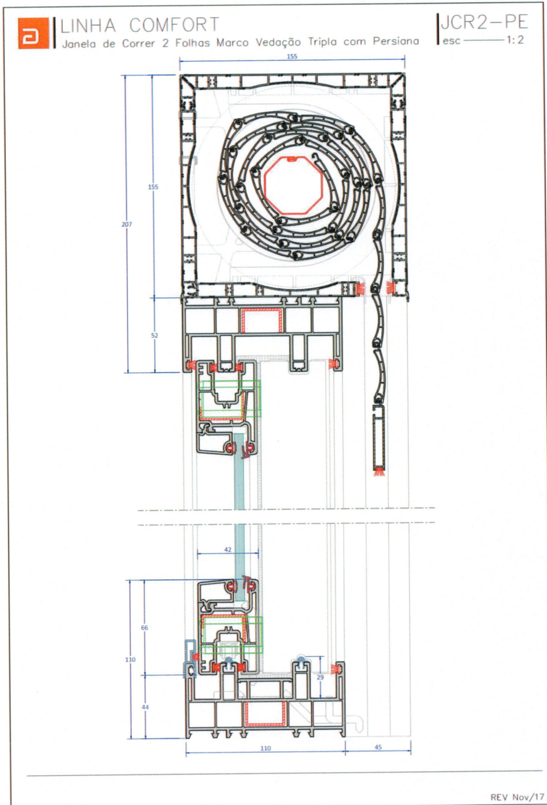
Figura – Projeto da esquadria com vidro 6 mm (TE-014, parte 1/2)
