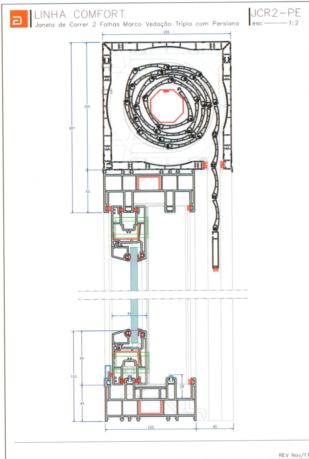
Figura – Projeto da esquadria com vidro laminado 5+5 mm (TE-015, parte 1/2)
