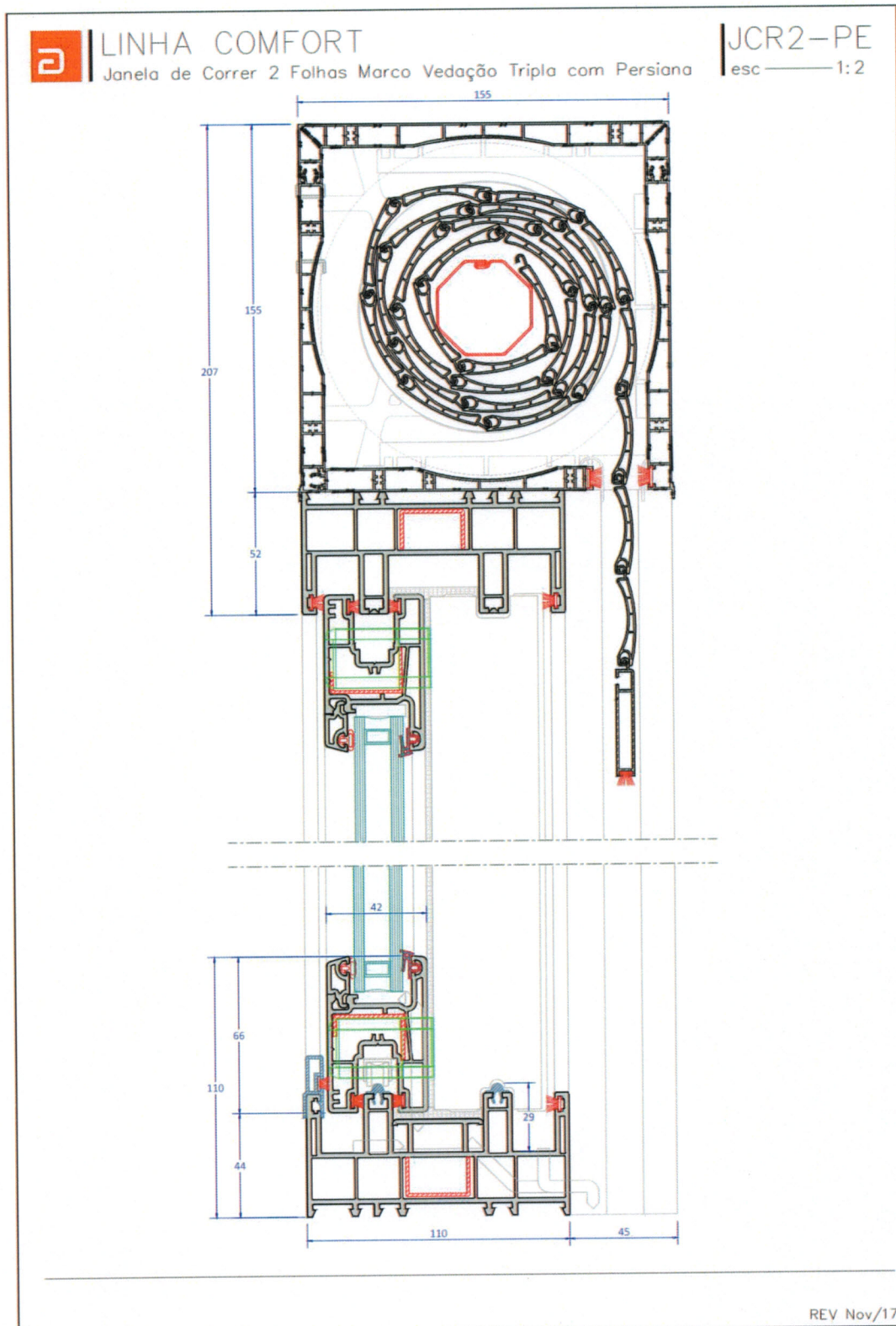
Figura – Projeto da esquadria com vidro insulado duplo de 10 mm e 4 mm (TE-016, parte 1/2)
