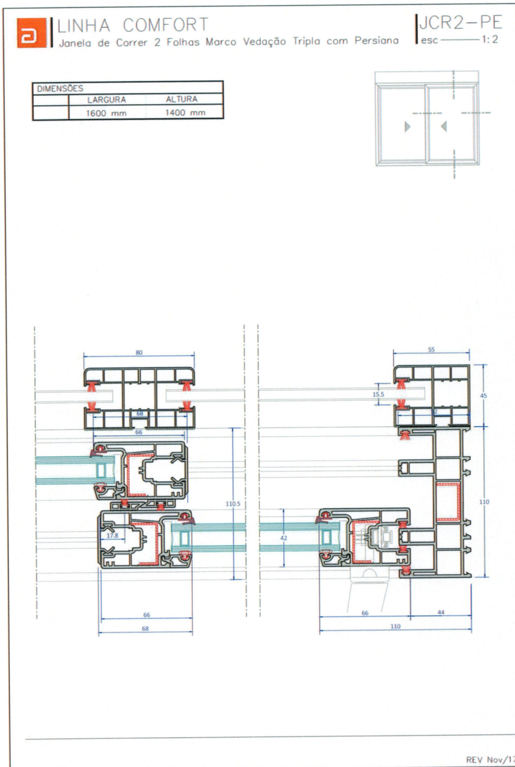
Figura – Projeto da esquadria com vidro insulado duplo de 10 mm e 4 mm (TE-016, parte 2/2)
