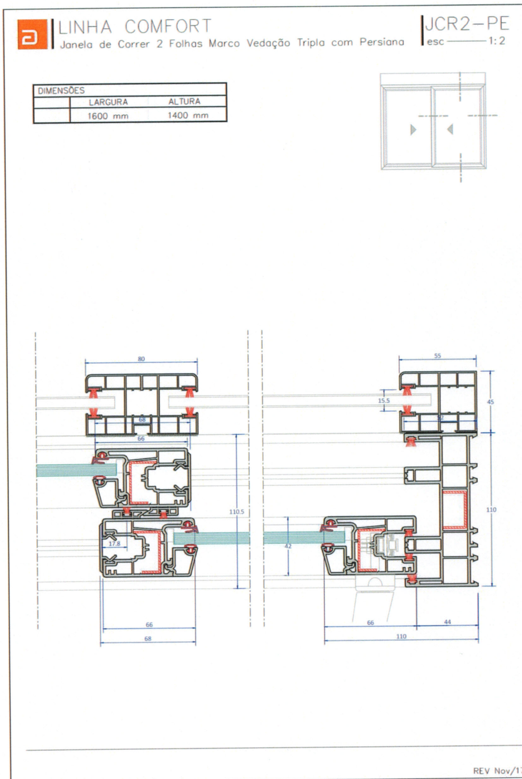
Figura – Projeto da esquadria com vidro laminado 5+5 mm (TE-015, parte 2/2)
