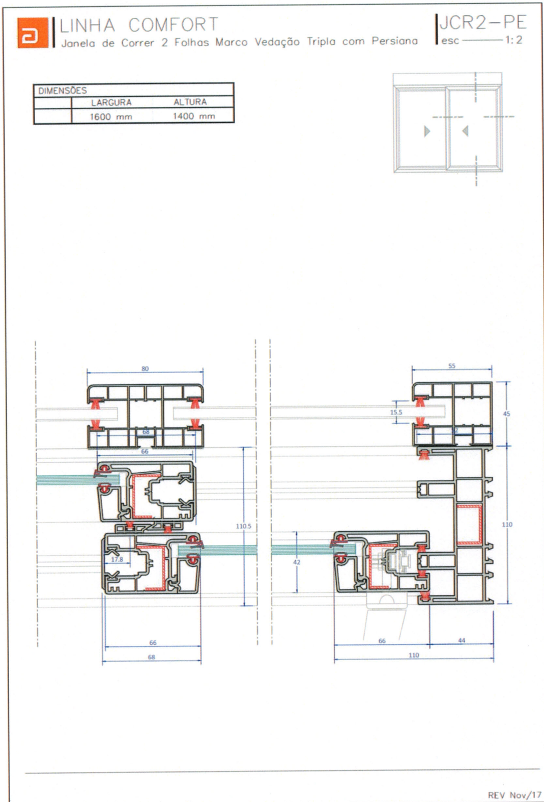
Figura – Projeto da esquadria com vidro 6 mm (TE-014, parte 2/2)
